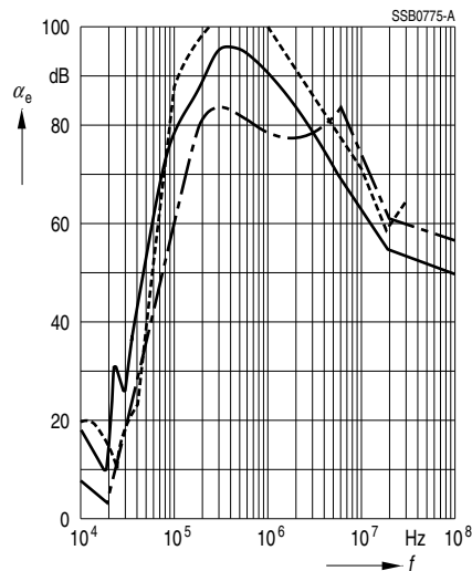
B84142-B16-R
